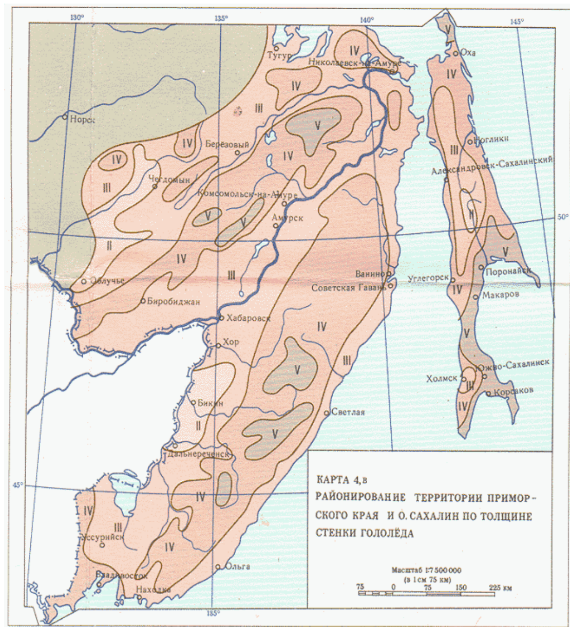
Карта 4, в Районирование территории Приморского Края и о. Сахалин по толщине стенки гололеда
