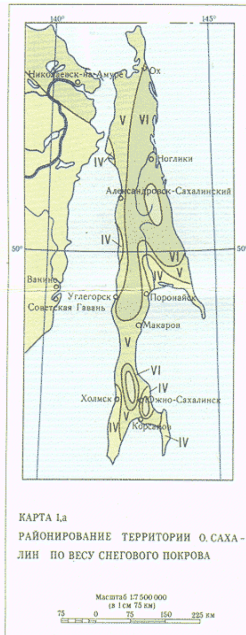
Карта 1, а Районирование территории о. Сахалин по весу снежного покрова
